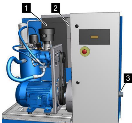
Рис. 21: Охладитель
