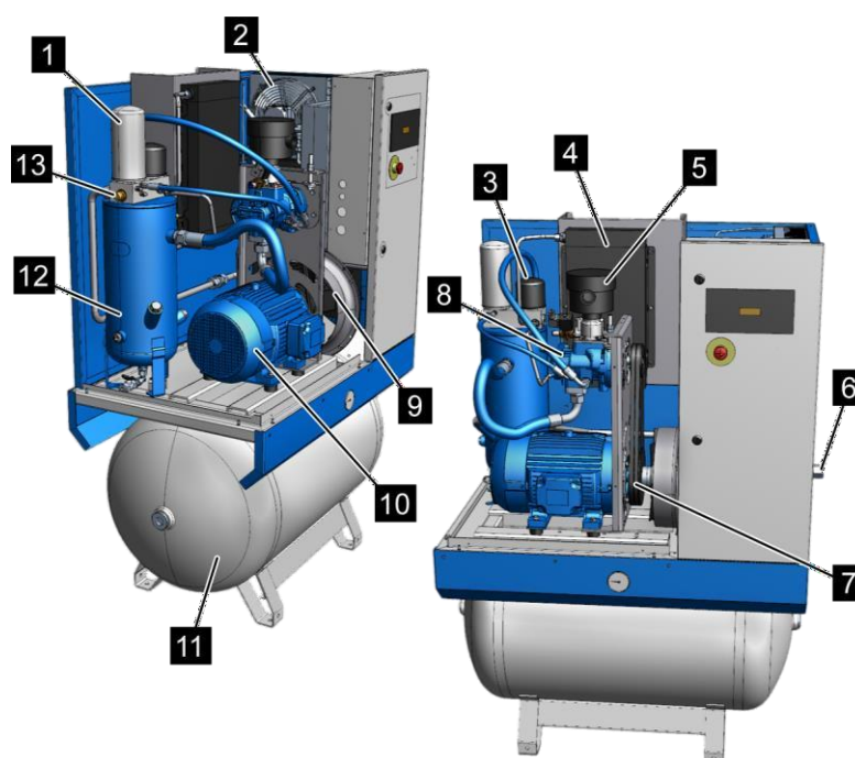
Рис. 10: Узлы типа 6 – 22
