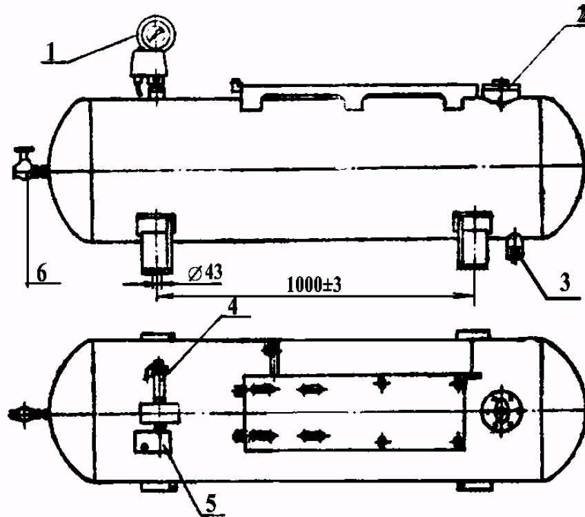
Рис. 20. Ресивер установки компрессорной, модель К-22
