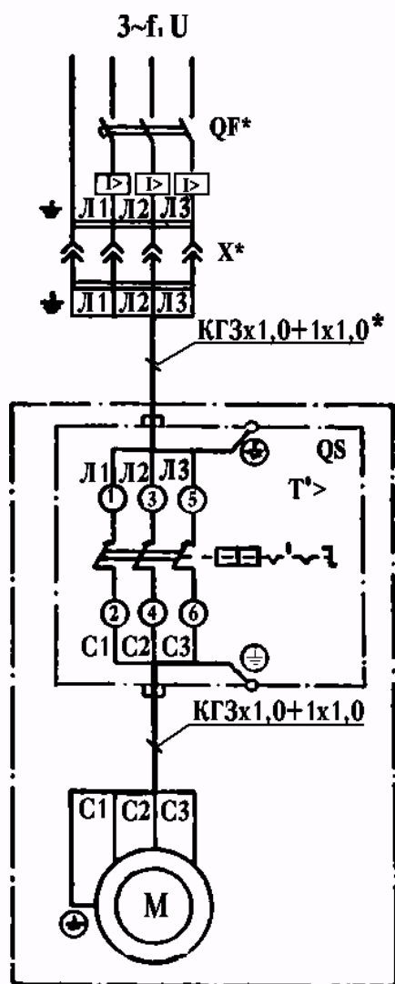
Рис. 33. Схема электрическая принципиальная и соединений установки компрессорной, модель K-2
