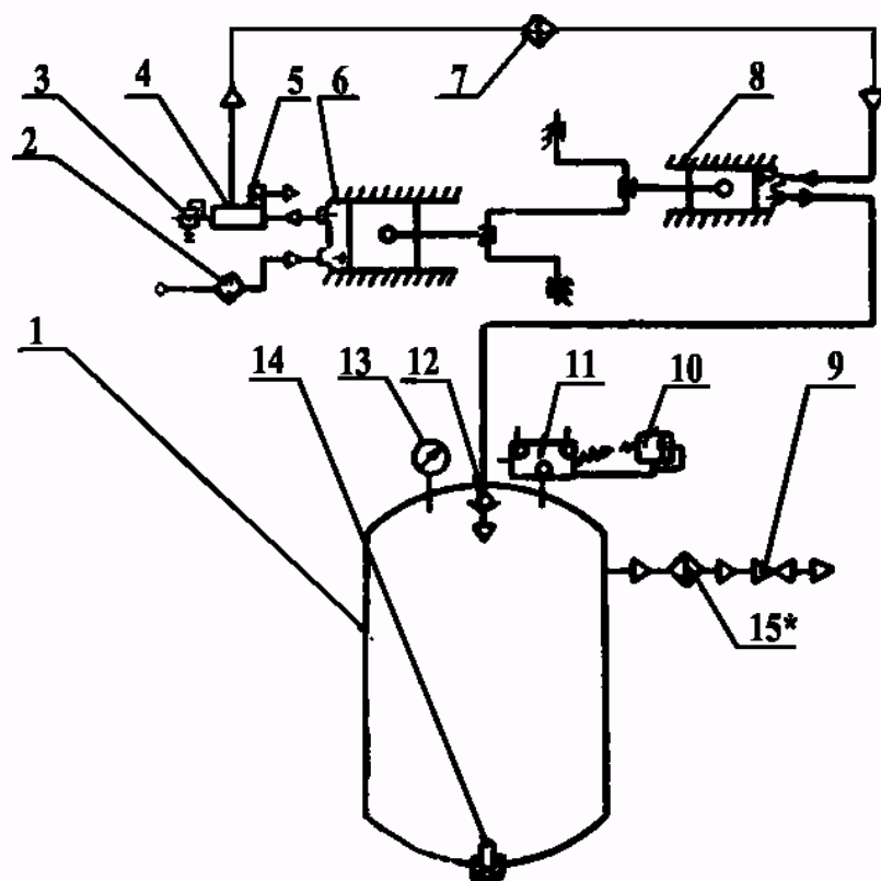
Рис. 32. Схема пневматическая принципиальная установки компрессорной, модель KV-15
