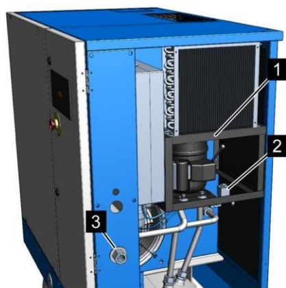
Рис. 23: Рефрижераторный осушитель
